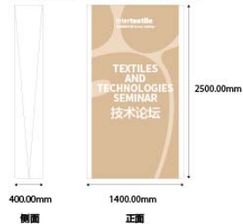
舞台两侧挂布结构和尺寸
